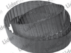
Código: P121 Nº Part: 094A910840 Máquina(s): Roland Pratica 00/01 Descrição: Correia sincronizada do motor principal
