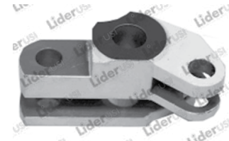
Código: P141 N° Part: 005A433230 Máquina(s): Roland Pratica 00 Descrição: Alavanca do rolete
