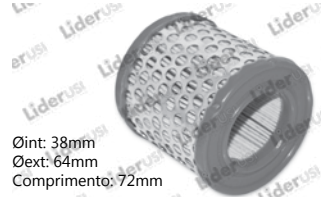
Código: P197 Nº Part: 350283 Máquina(s): Roland Pratica 00/01 Descrição: Filtro p/ compressor menor
