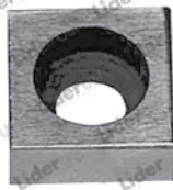
Código: P293 Nº Part: 006E096230 Máquina(s): Roland Pratica 00/01 Descrição: Calço da alavanca do trinquete
