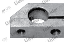
Código: P312 Nº Part: 010C162830 Máquina(s): Roland Pratica 00/01 Descrição: Corpo da pinça
