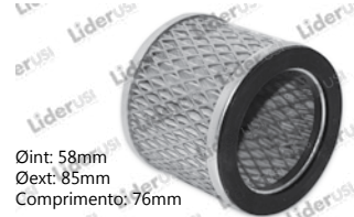
Código: P197A Nº Part: 350273 Máquina(s): Roland Pratica 00/01 Descrição: Filtro p/ compressor maior
